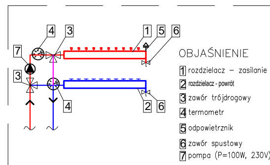
Szczegóły A Rozdzielacz z mieszaczem pompowym
